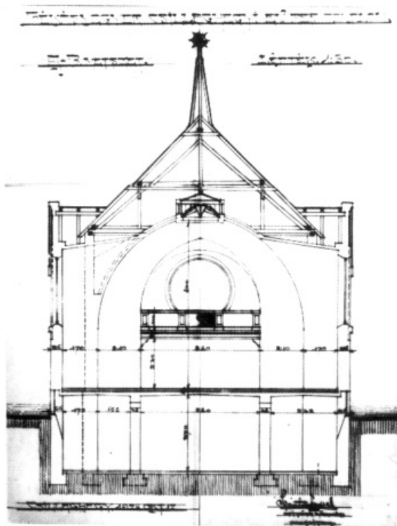
Csillaghegy, református templom terve, keresztmetszet. 1928.
