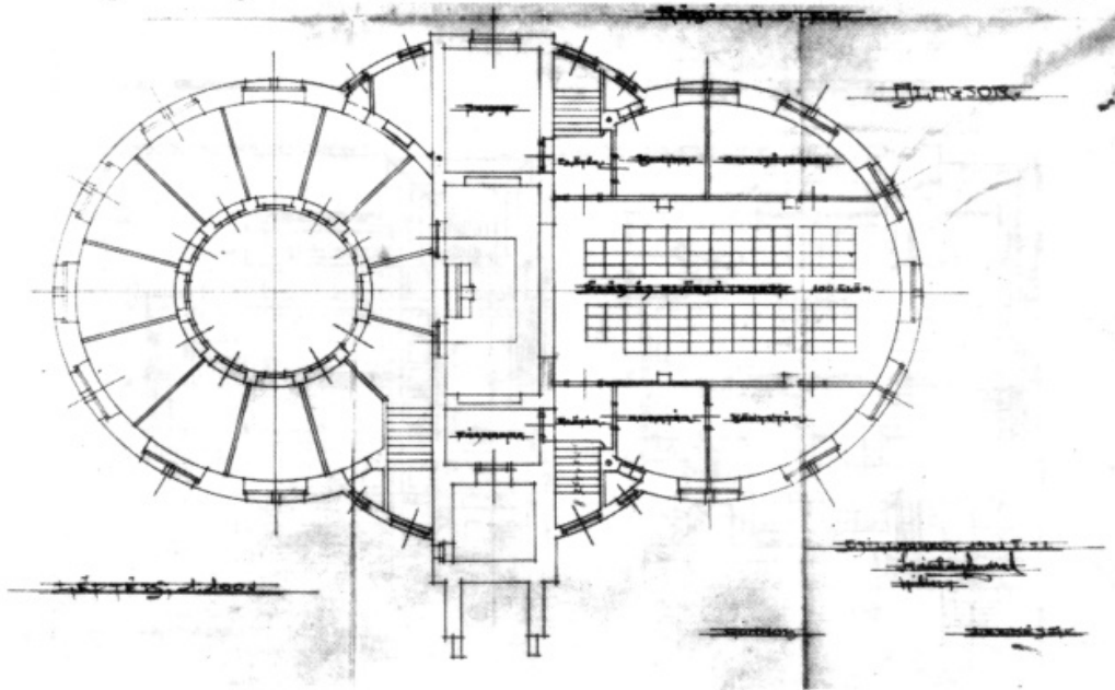
Csillaghegy, református templom, II. sz. terve alagsori alaprajz. 1931. Balra: Református Pantheon, jobbra: Előadóterem
