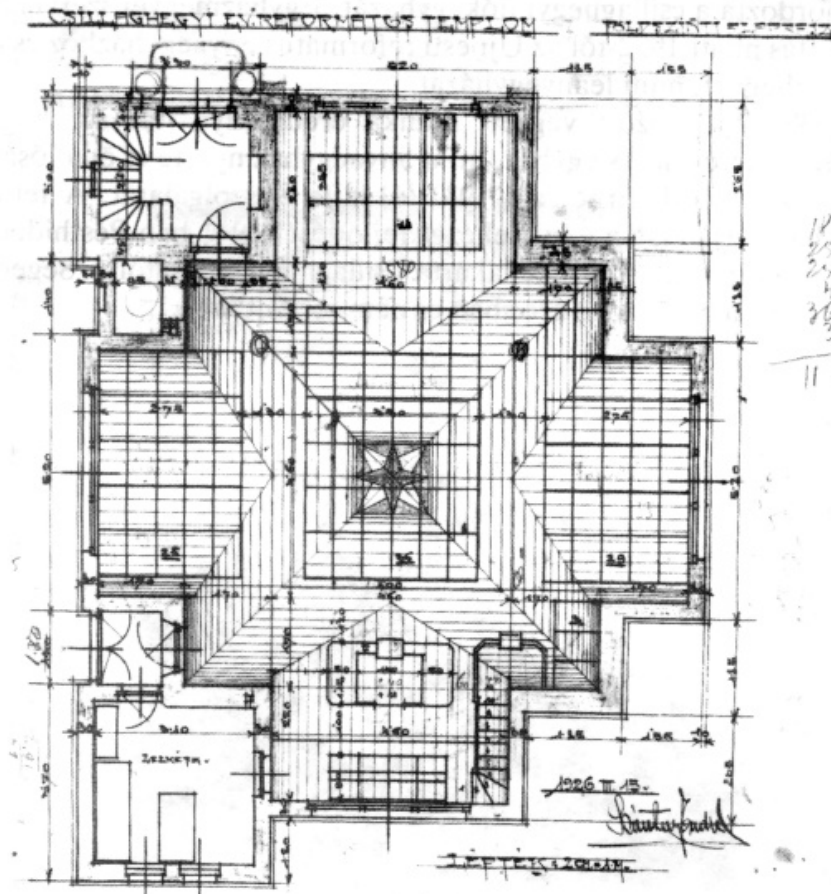
Szántay Endre: Csillaghegy, református templom alaprajzi terve. 1926.
