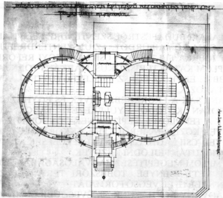
A csillaghegyi református templom II. számú terve. 1931. Földszinti alaprajz.
