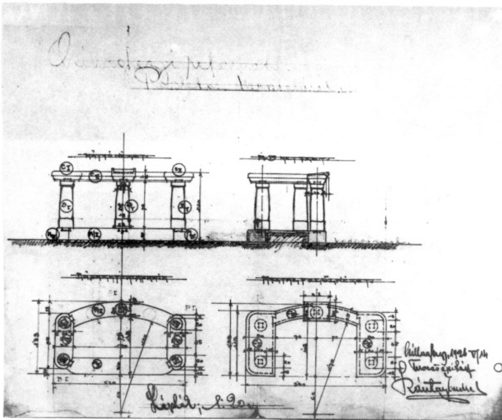
Csillaghegy, református templom Úr Asztal terve. 1926.
