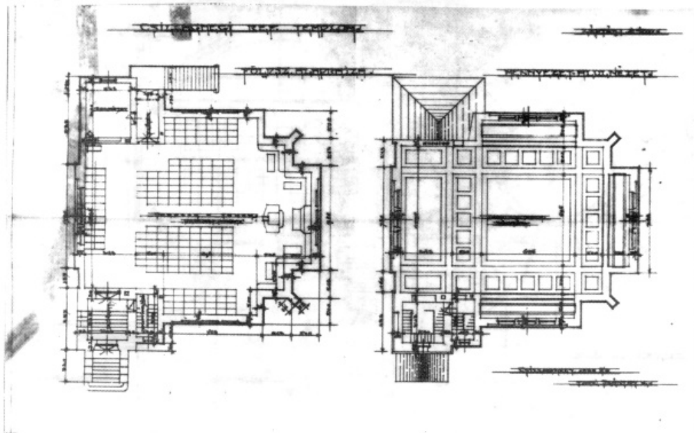
Szántay Endre: Csillaghegy, református templom, földszinti alaprajz és mennyezet alulnézete. 1936.
