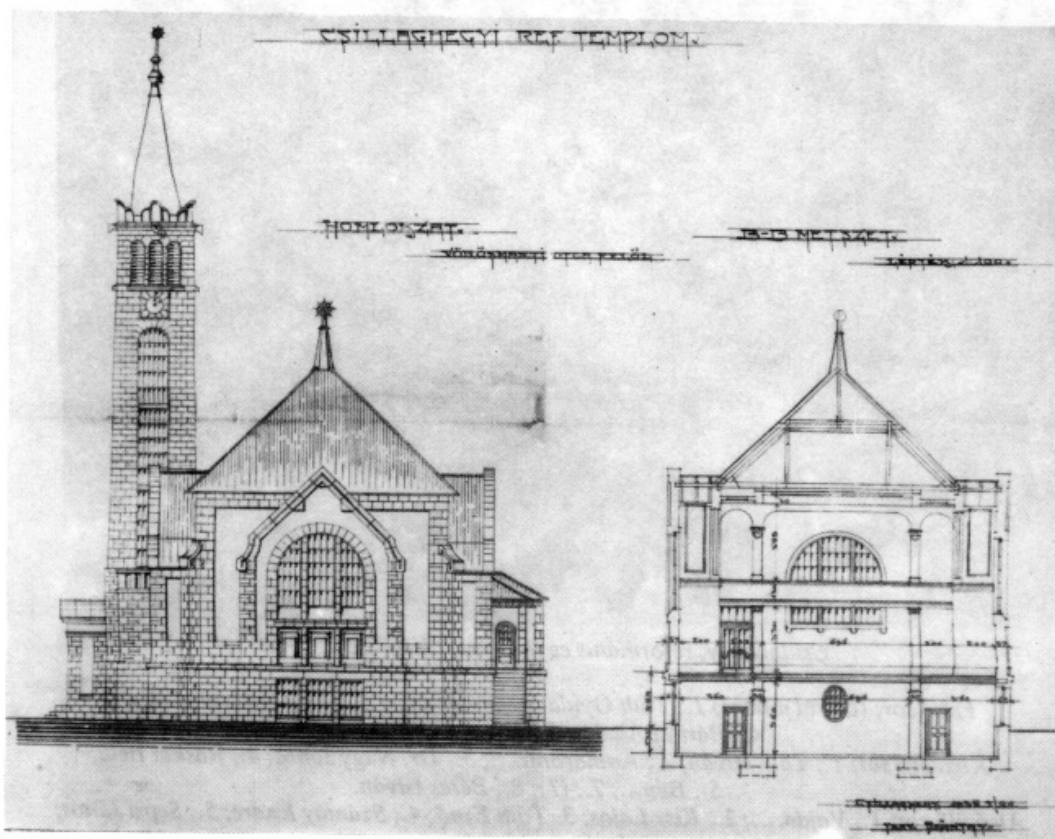
Szántay Endre: Csillaghegy, református templom terve, oldalhomlokzat és metszet. 1935.
